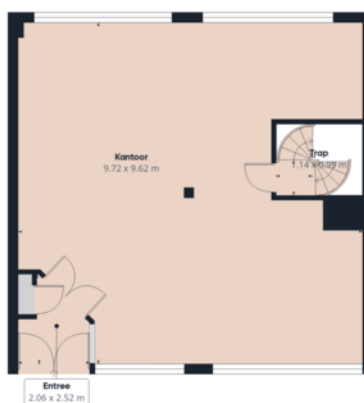
Etage 0
